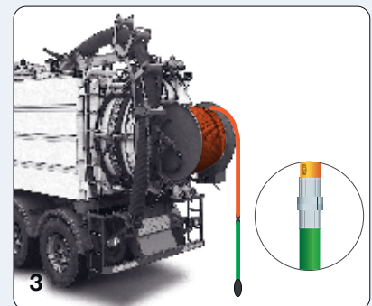
Rubber or thermoplastic "Leader Hose"; to facilitate the operation and to signal the nozzle return. Tubo Leader di gomma o termoplastico che faciliti l'operazione di inserimento e segnali l'uscita dell'ugello durante il recupero del tubo.
